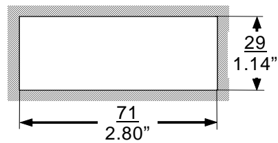
Fig. 5 Découpe du panneau
