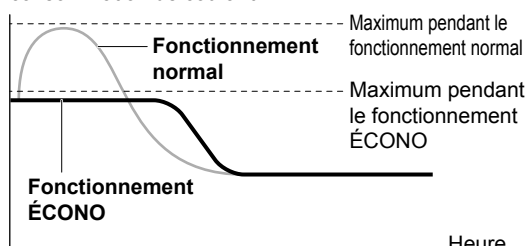
Courant de fonctionnement et consommation de courant
